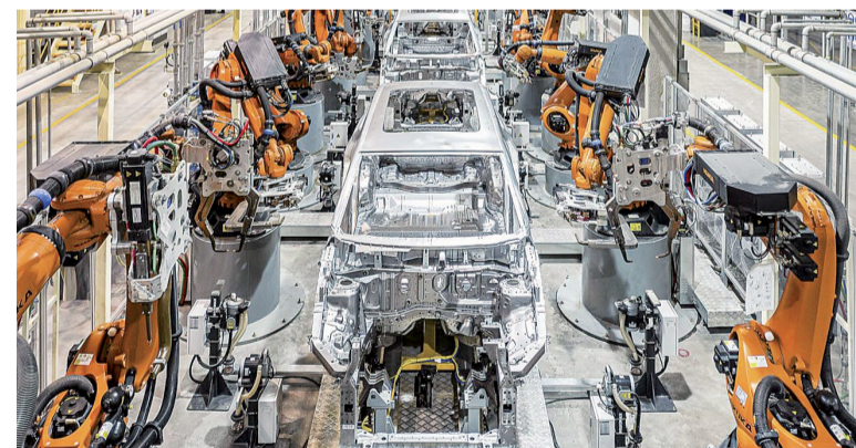
长安汽车生产线
