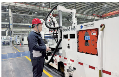
中国煤科重庆研究院钻探分院研发的“智钻先锋”机器人 陈军 摄
